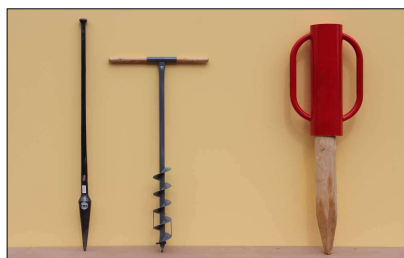
Werkzeuge zum Versetzen der Rundsteher
